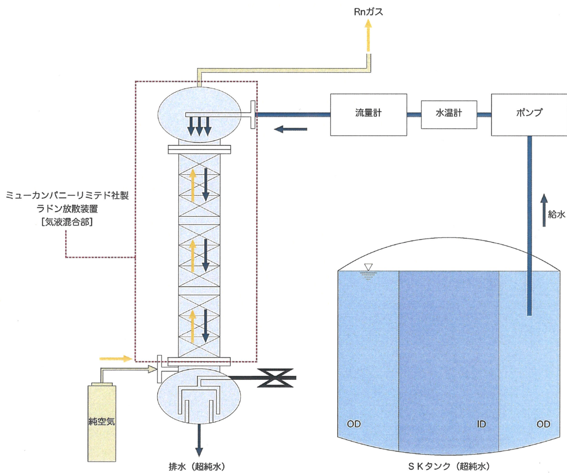
SK純水中ラドン濃度測定装置 [部分]
