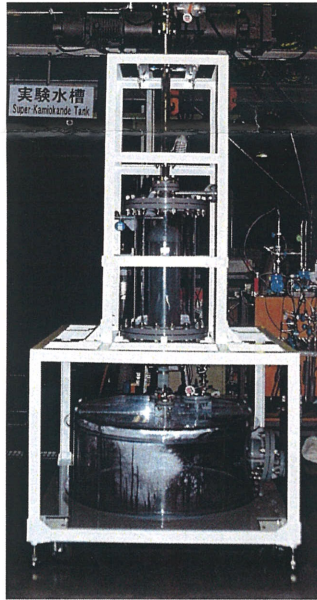
ラドン放散装置
